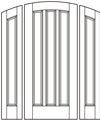
NHF 94231BVI & 9423SBVI 1'2" + 3'0" + 1'2" x 6'8" x 1 3/4"
